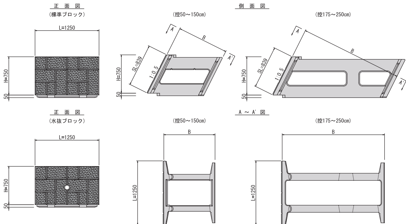
大型ブロック 製品規格表 (控長35~150cm)
