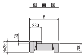
基礎ブロック 製品規格表 (控長35~75cm)
